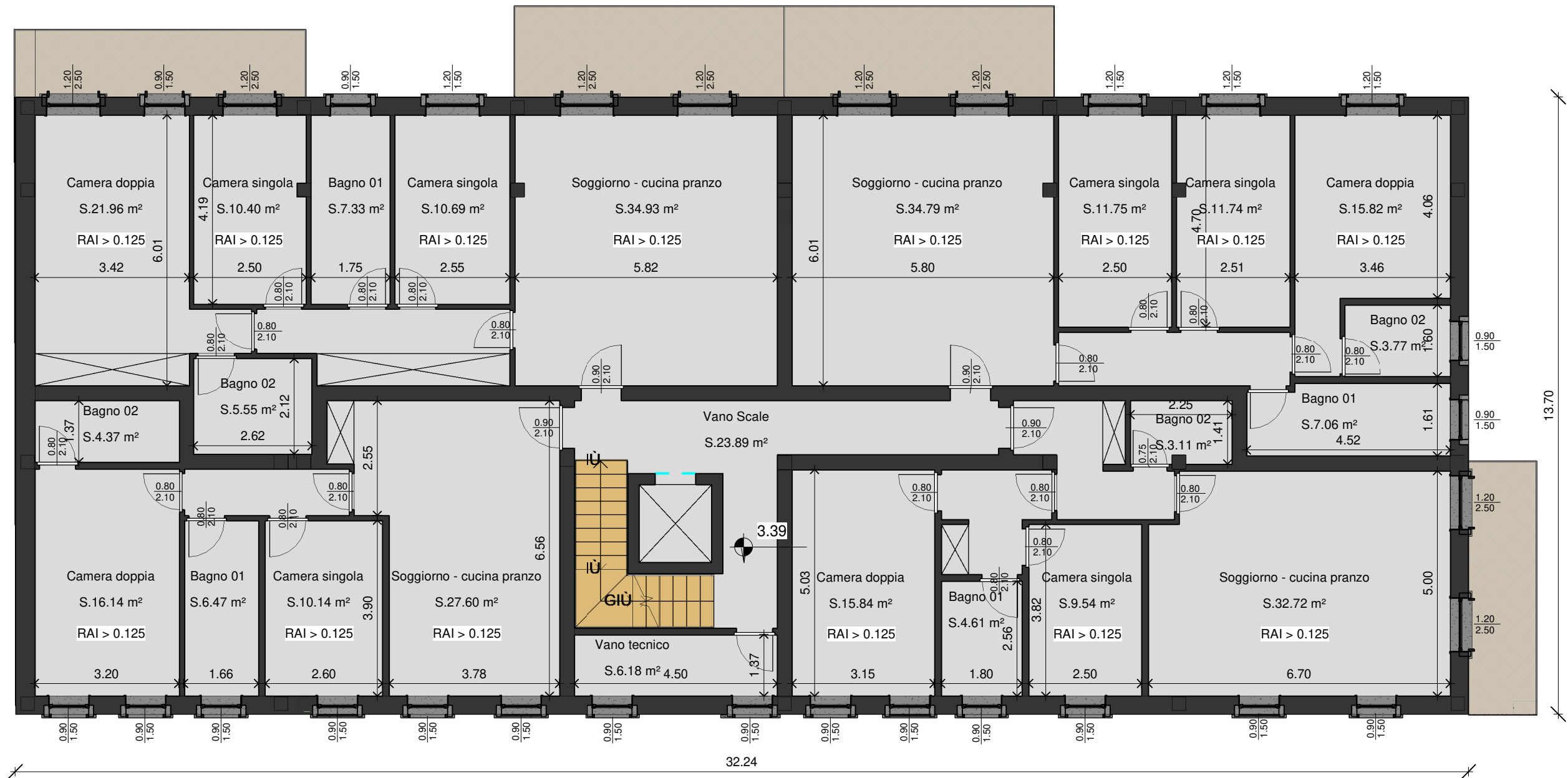
PIANO PRIMO 1.100
